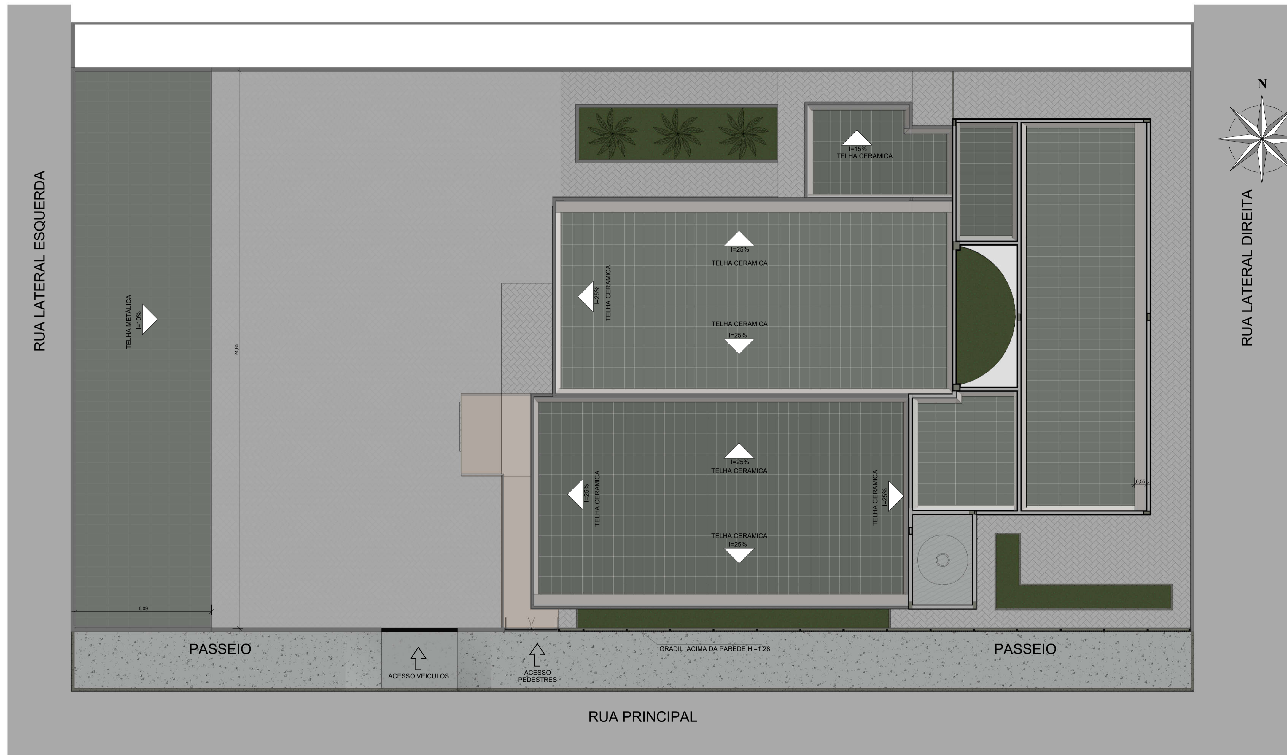
1 PLANTA DE COBERTURA - FINAL ESCALA 1:100
